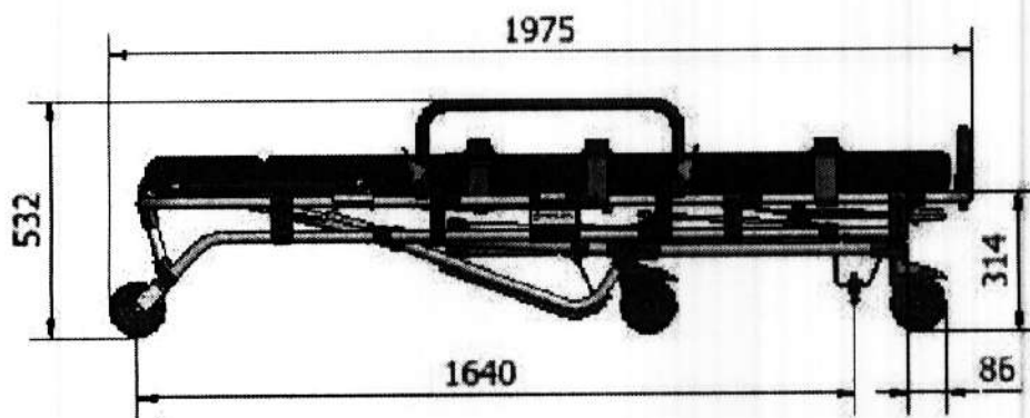
Figura 03 – Maca desarmada
