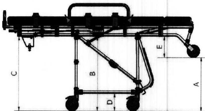
Figura 04 – Vista lateral
