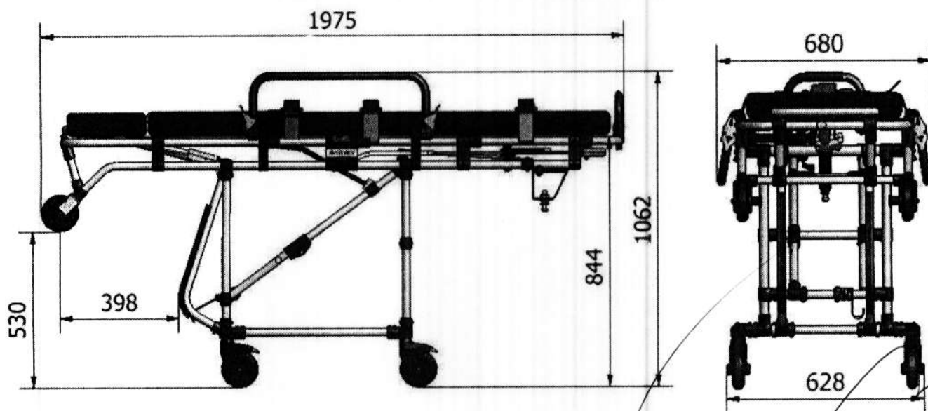
Figura 02 – Maca Armada
