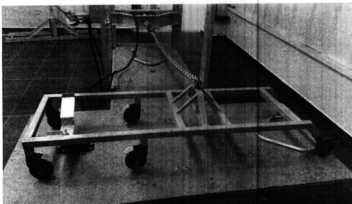
Foto 07-Aplicação de carga no sentido lateral
